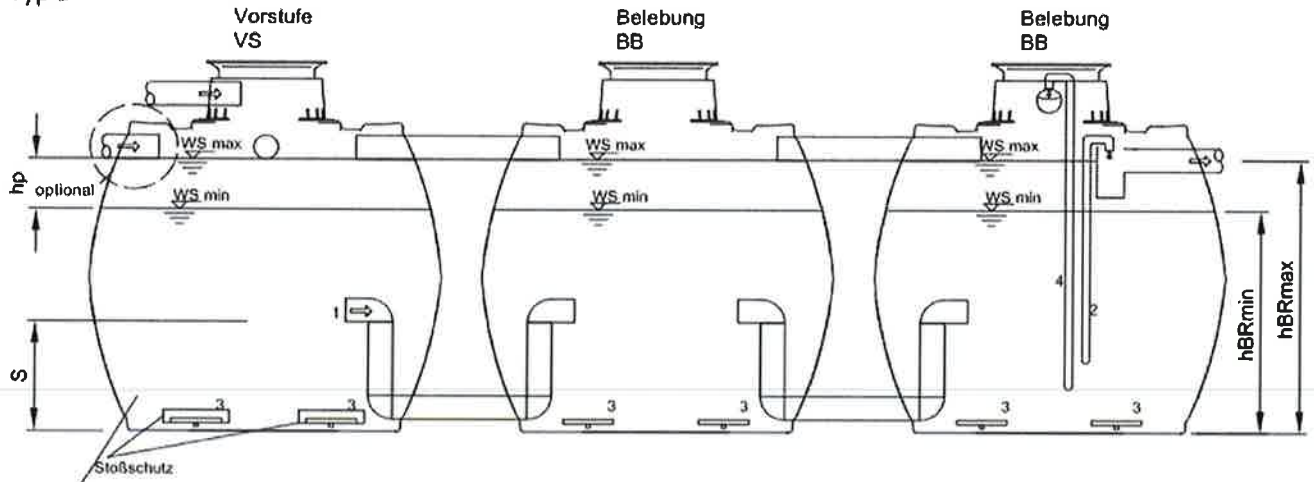
Entschlammungskammer
